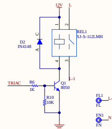
加热线电路
